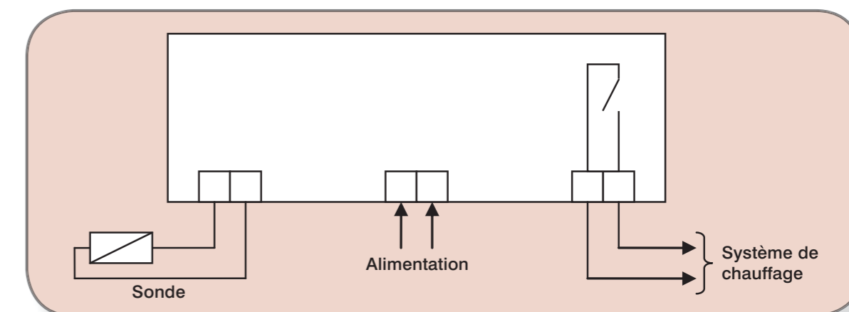
Figure 3 : Schéma électrique d'un thermostat standard
